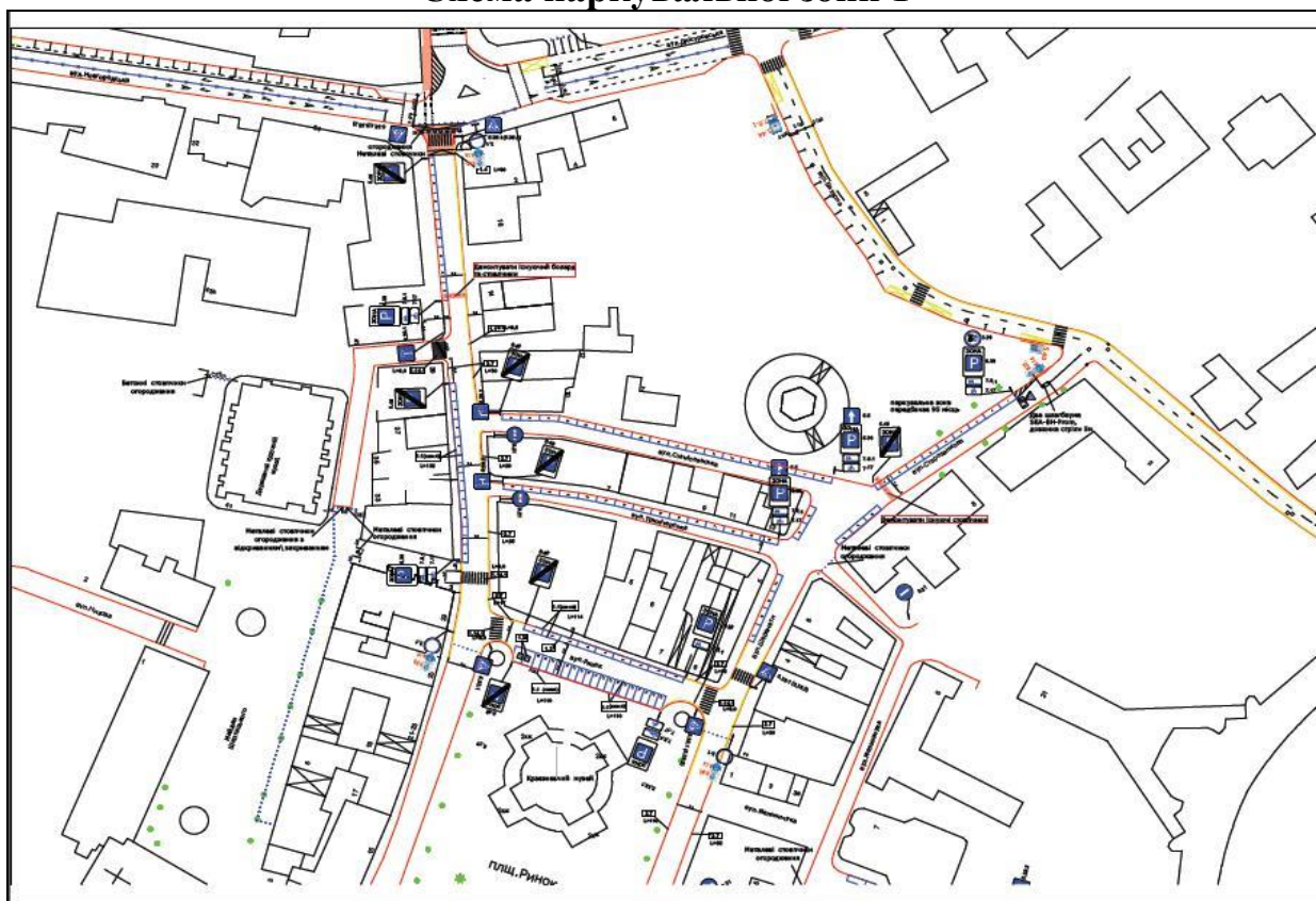
Схема паркувальної зони 1
